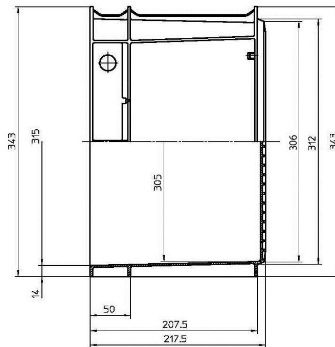
断面図
