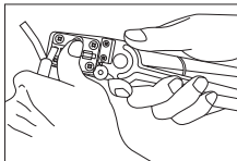
③親指を指あてにあて先端で芯線の皮を剥く。
