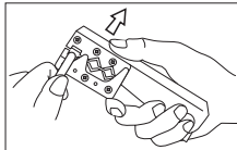
②先端の刃で芯線の絶縁部分を切り離す。
