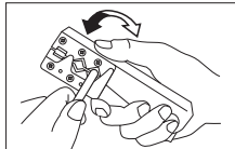
①同軸ケーブルを刃で挟む(5Cは上刃、JISその他は下刃)。刃を前後に180°回転させて動かし、外皮を剥く。
