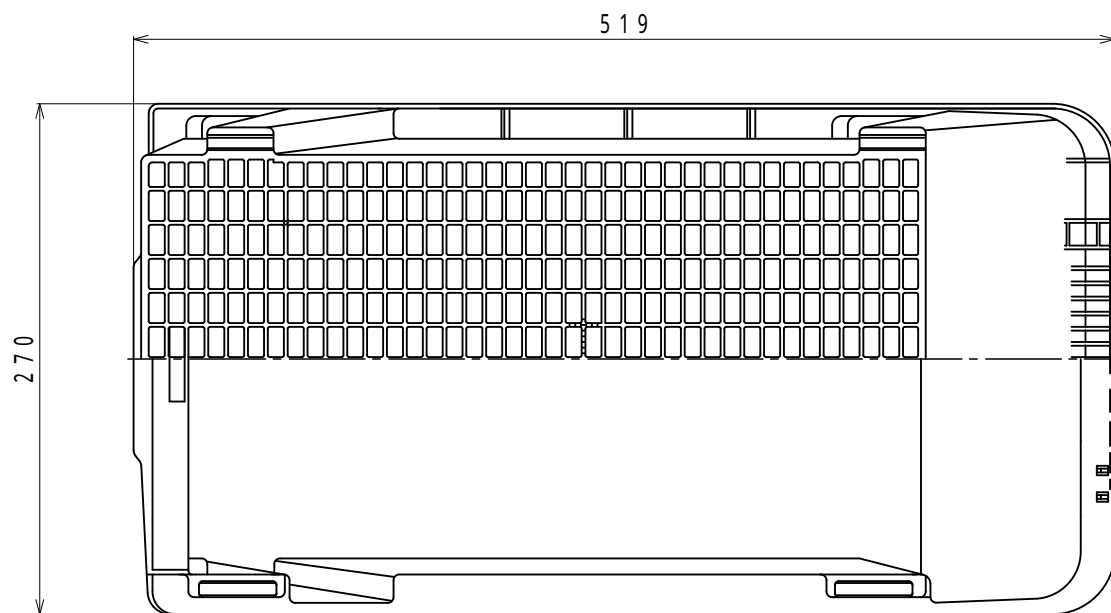
平面図 / 底面図
