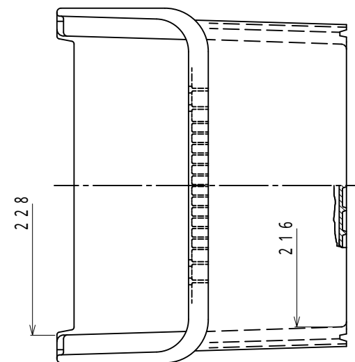
正面図 / 断面図
