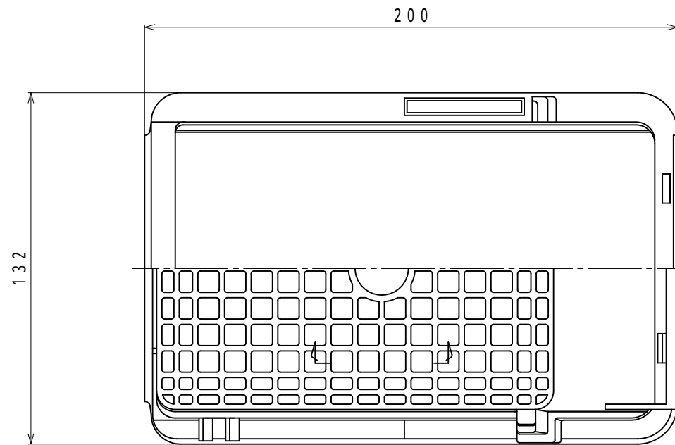
平面図 / 底面図
