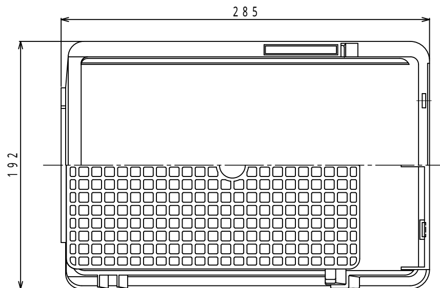
平面図 / 底面図
