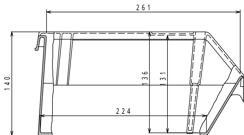
側面図 / 断面図
