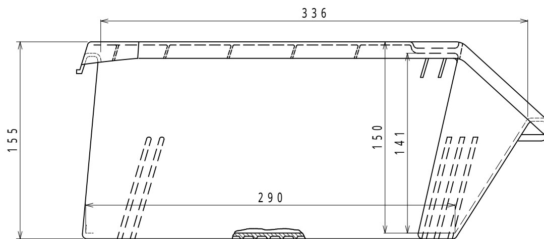
側面図 / 断面図
