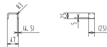
フック詳細
