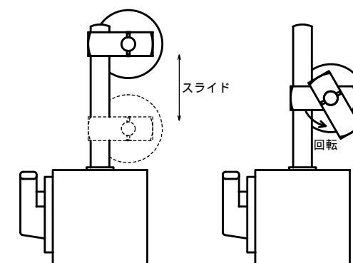
動作図 (縮尺 1:2)
