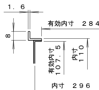
A-A断面 (S=1:2)
