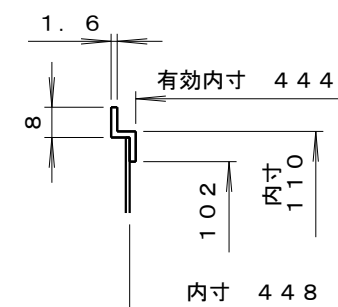
B-B断面 (S=1:2)
