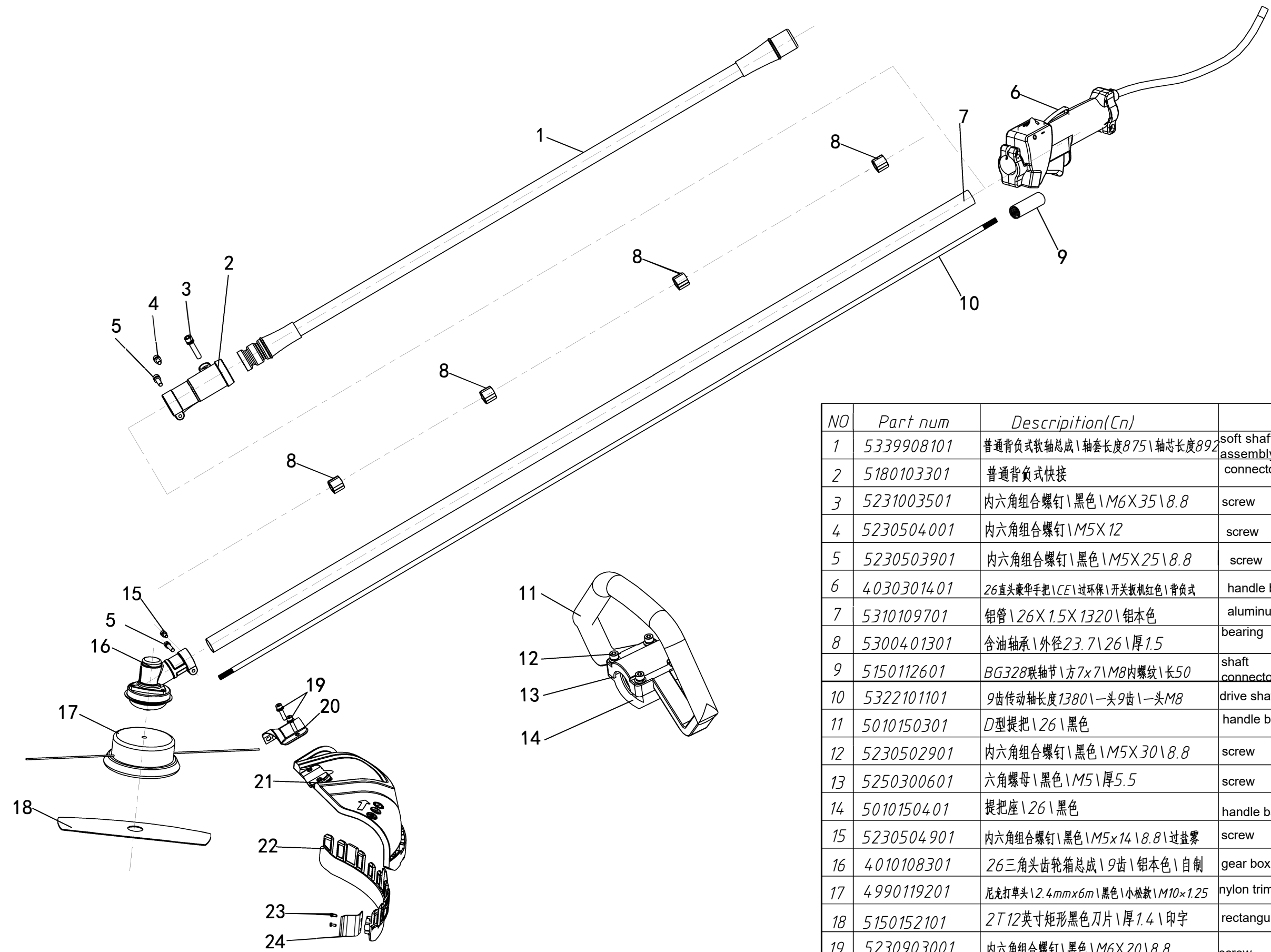
杆子爆炸图
