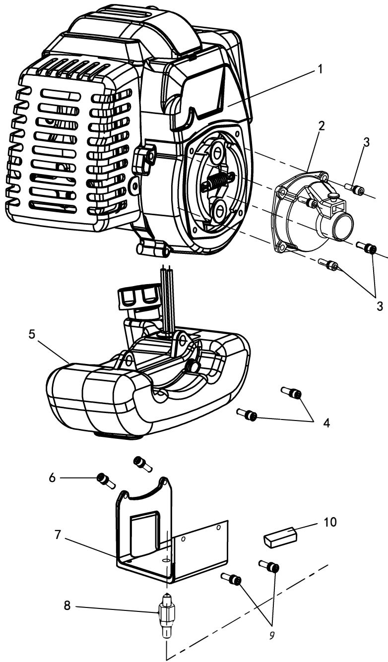
低背架爆炸图
