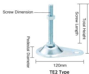
TE2 Type (steel)
