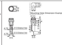
Dimensions (F-240-N)
