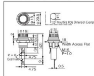
Dimensions (F-120-B)
