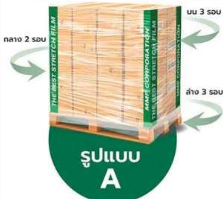
พาเลทวางสินค้าทั่วไป จำพวกคลัง (แบบเสมอพาเลท)
