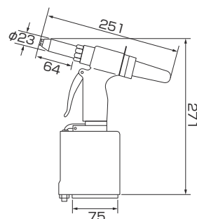
寸法図 AR011MX
