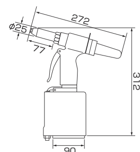
寸法図 AR011HX
