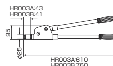
寸法図 HR003A・B
