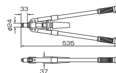
寸法図 HR2050H
