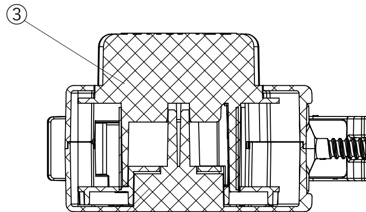
断面図 B-B
