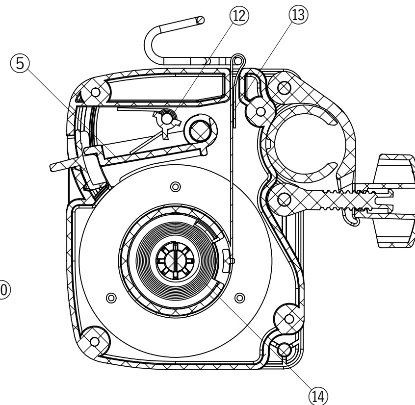
断面図 A-A
