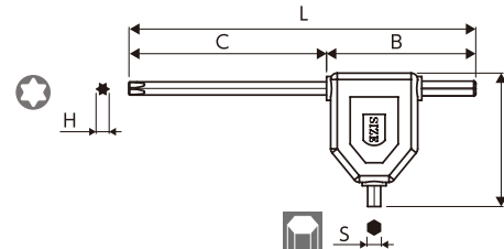
精密ヘックスローブレンチセット フラッグタイプ【6本入り】※同サイズが6本入っています。
