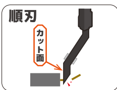
ディスクリード足切断
