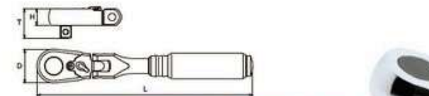
3726Z 首振りラチェットハンドル PATENTED
