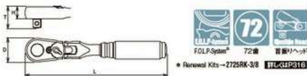
2726Z-3/8 (L160) 1/4" (6.35mm) SQ.のロングラチェットボディに3/8" (9.5mm) SQ.の差込角を設けたスリムタイプ。
