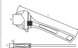
寸法図
