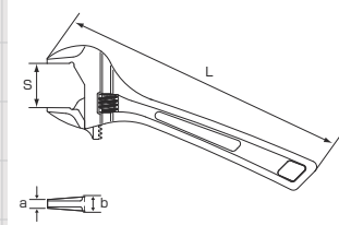
寸法図
