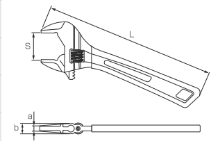
寸法図
