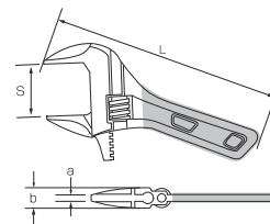
寸法図
