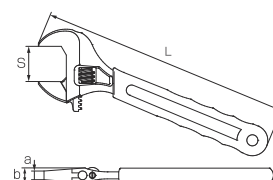
寸法図
