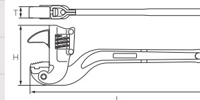
寸法図
