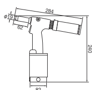
寸法図 AR2000SV
