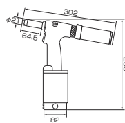
寸法図 AR2000MV
