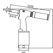
寸法図 AR2000HV
