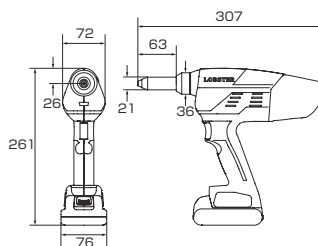
寸法図
