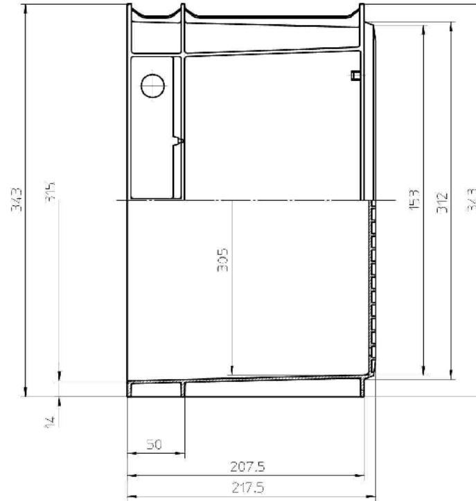
断面図
