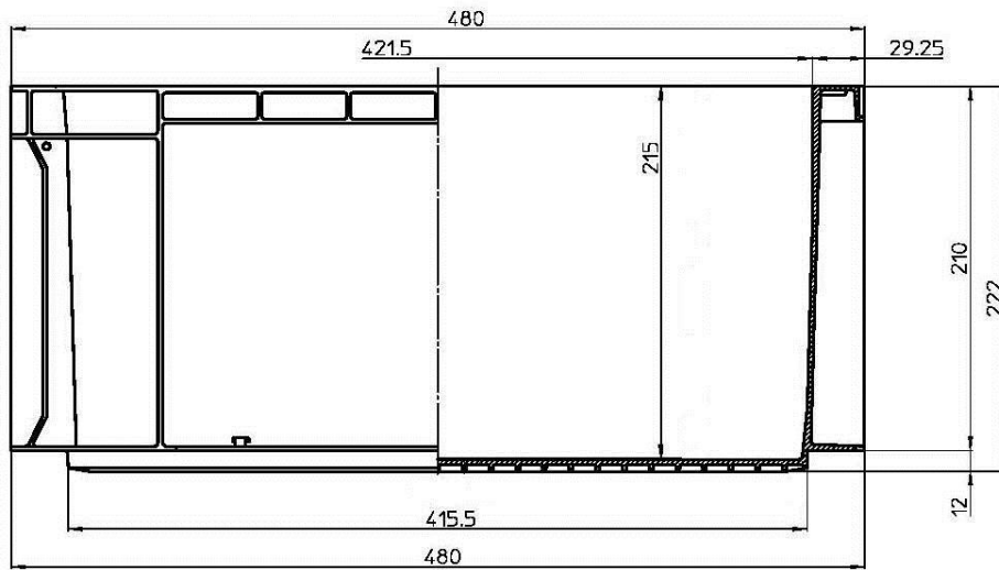
正面図
