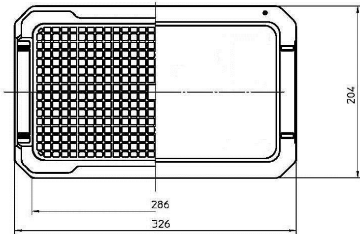
下面図
