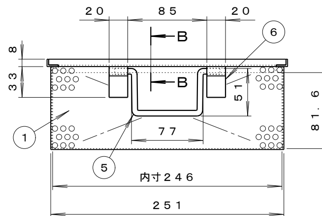
A-A断面 (S=1:2)
