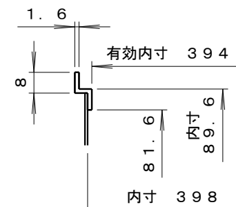
B-B断面 (S=1:2)
