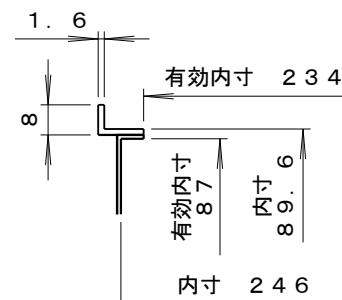
A-A断面 (S=1:2)
