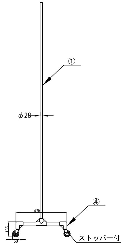
側面図
