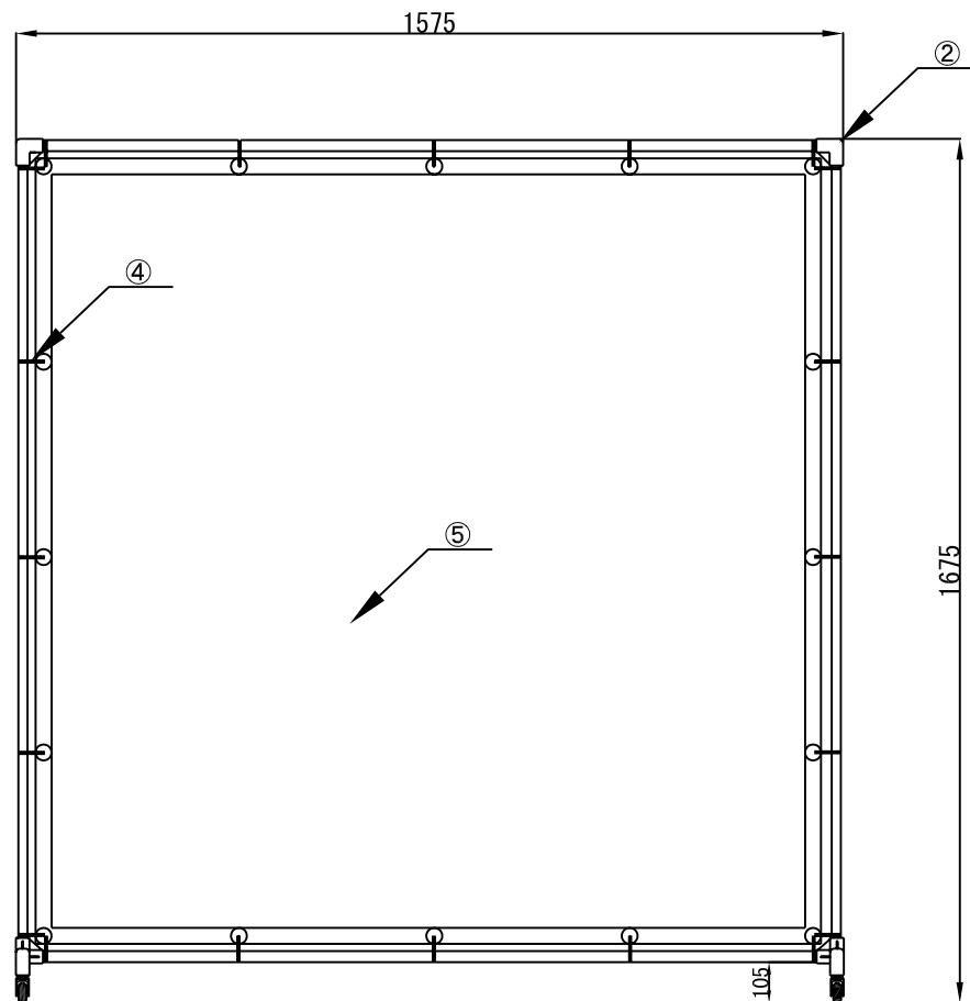
正面図
