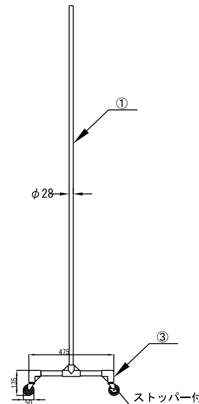
側面図
