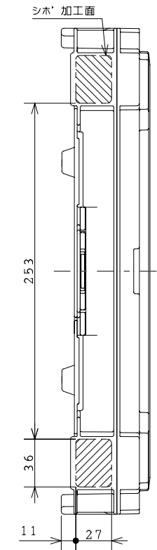
オリタタミ状態図
