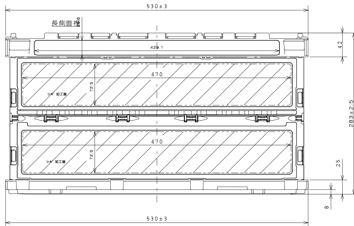
オリタタミ状態図
